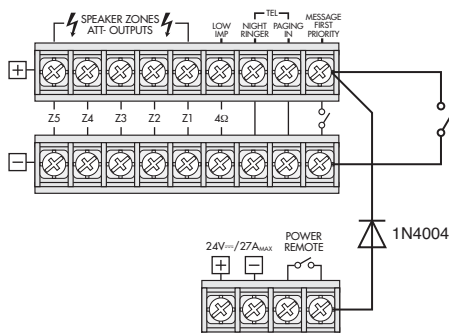
⑥ Conexión automática del amplificador y activación del anuncio M 6
